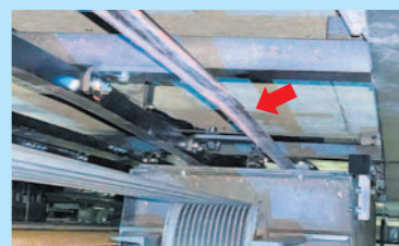
大・中ホール舞台吊物装置 昇降用レール変形
