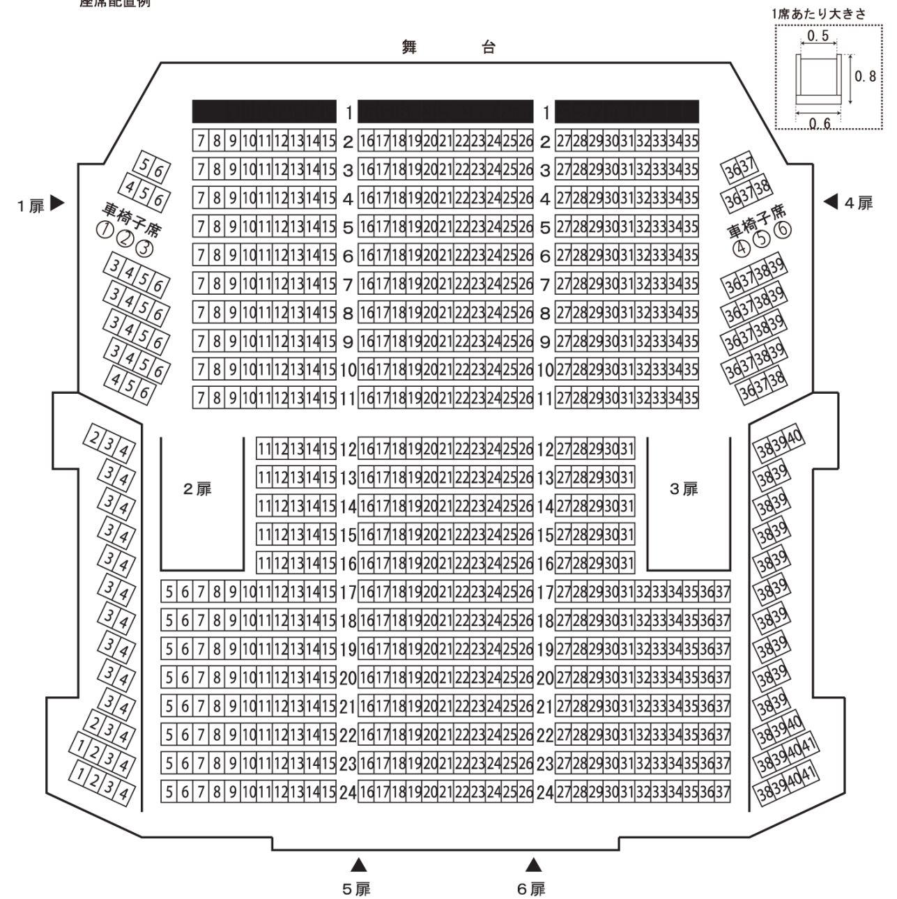
郡山市民文化センター中ホール座席配置図 単位:m 806席(うち車椅子席6席) □固定席771席・車椅子6席
