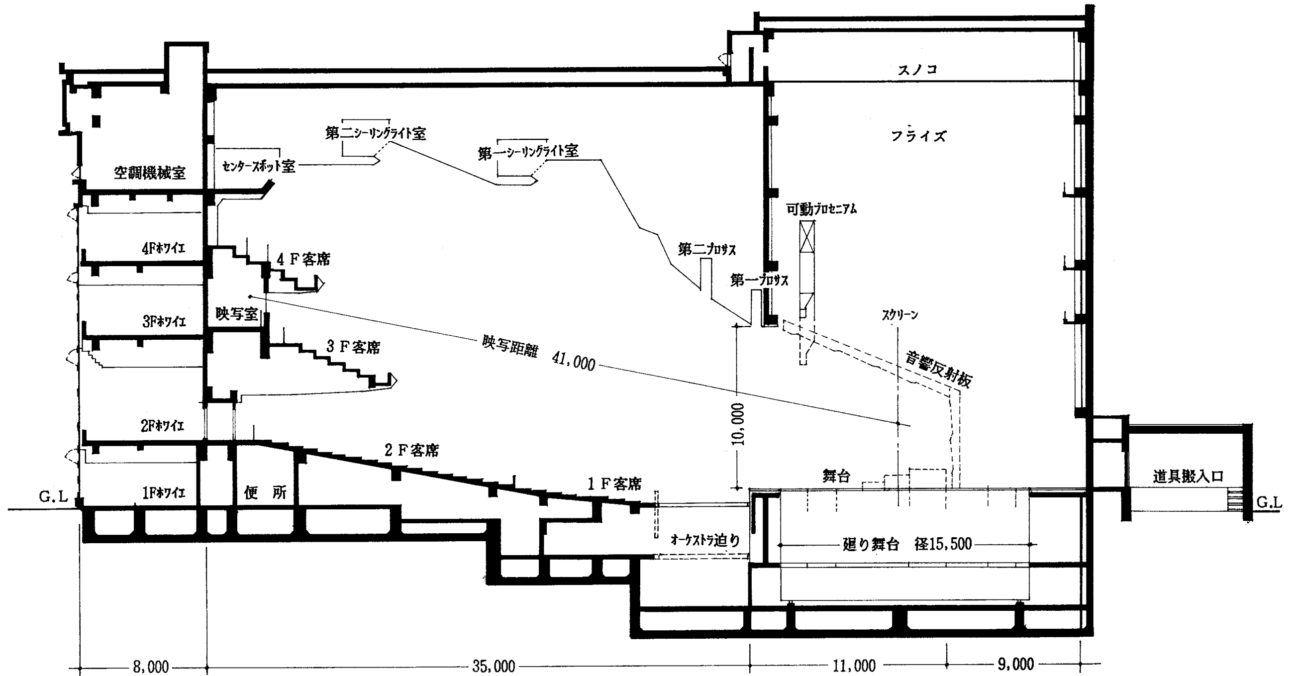
郡山市民文化センター 大ホール断面図
